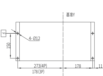
连接尺寸
