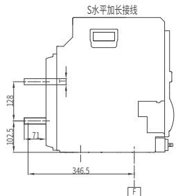
连接尺寸
