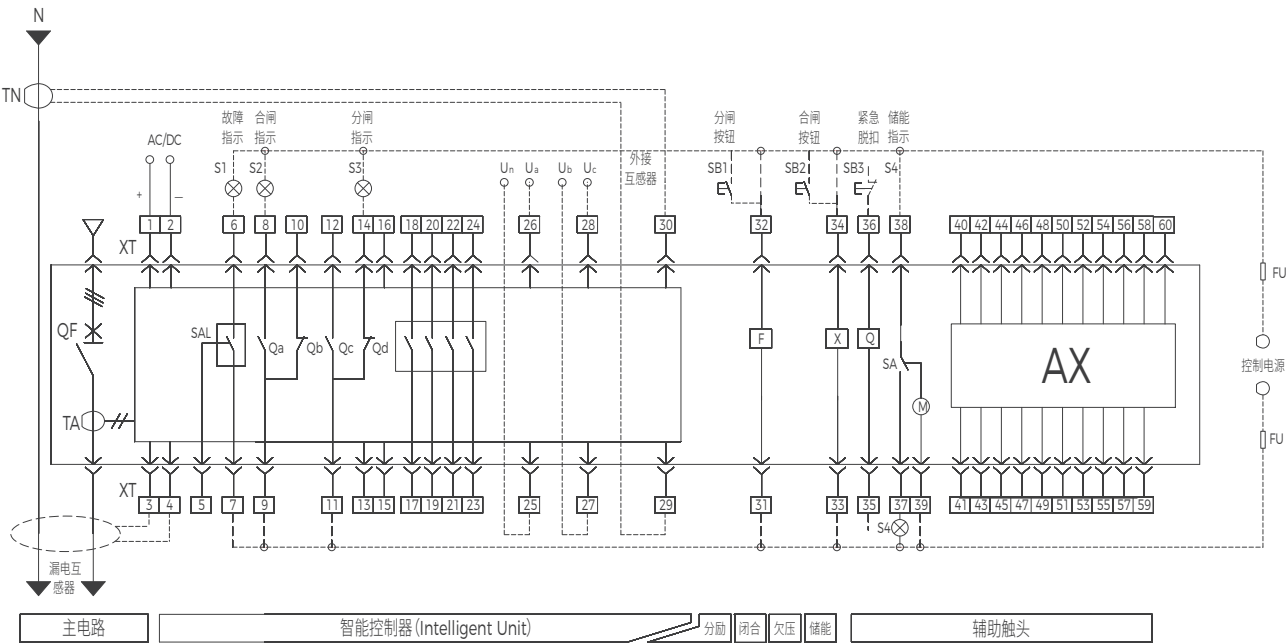
BW3-2500/3200/4000/5000/6300/8000 二次回路接线图
