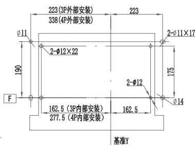
安装尺寸
