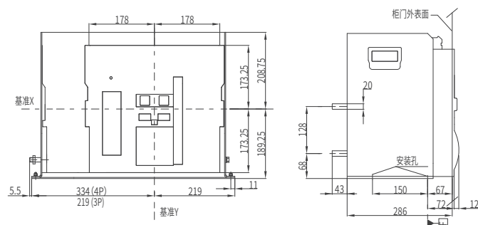
外形尺寸
