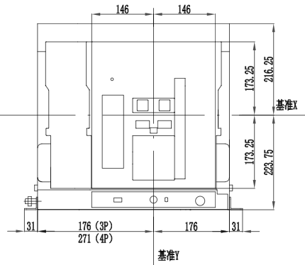
连接尺寸
