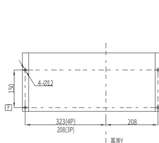
安装尺寸
