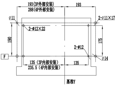
安装尺寸
