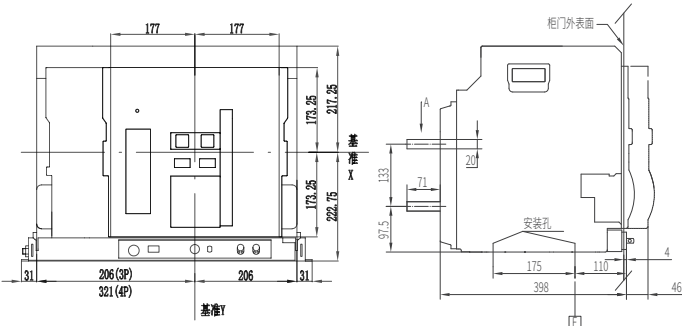
外形尺寸
