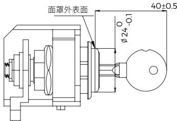
2000 壳架及以上钥匙锁外形尺寸
