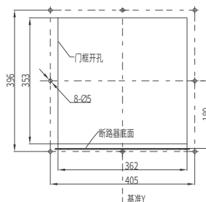
面板开孔尺寸
