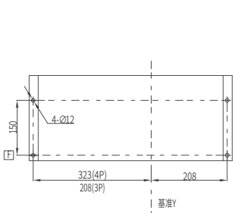
安装尺寸
