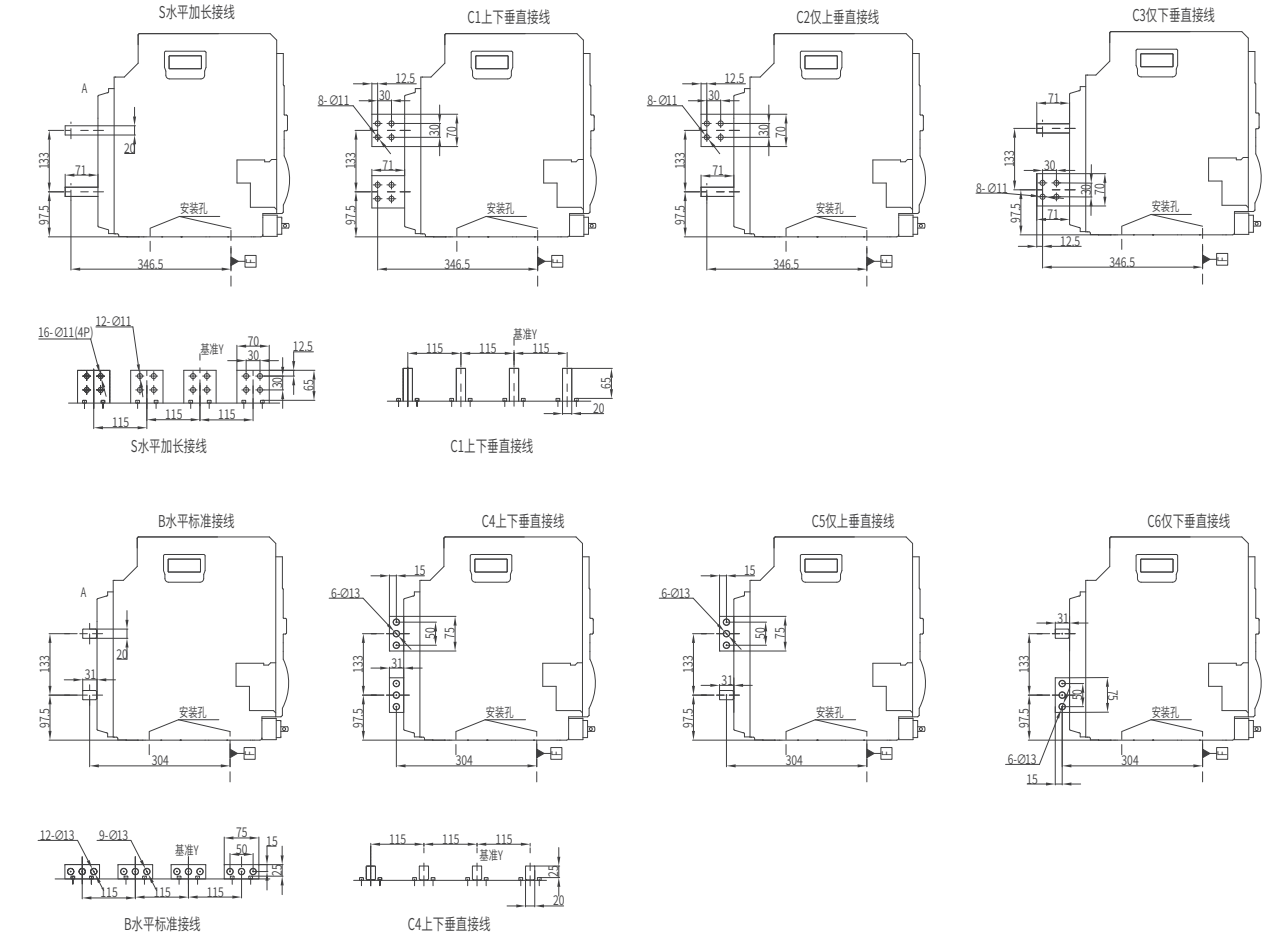
连接尺寸
