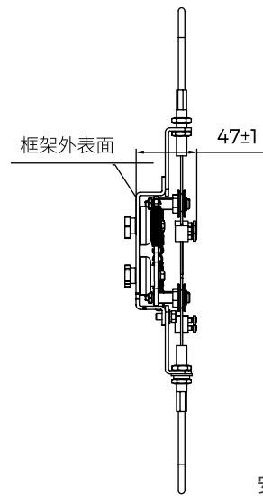
安装钢缆联锁外形尺寸
