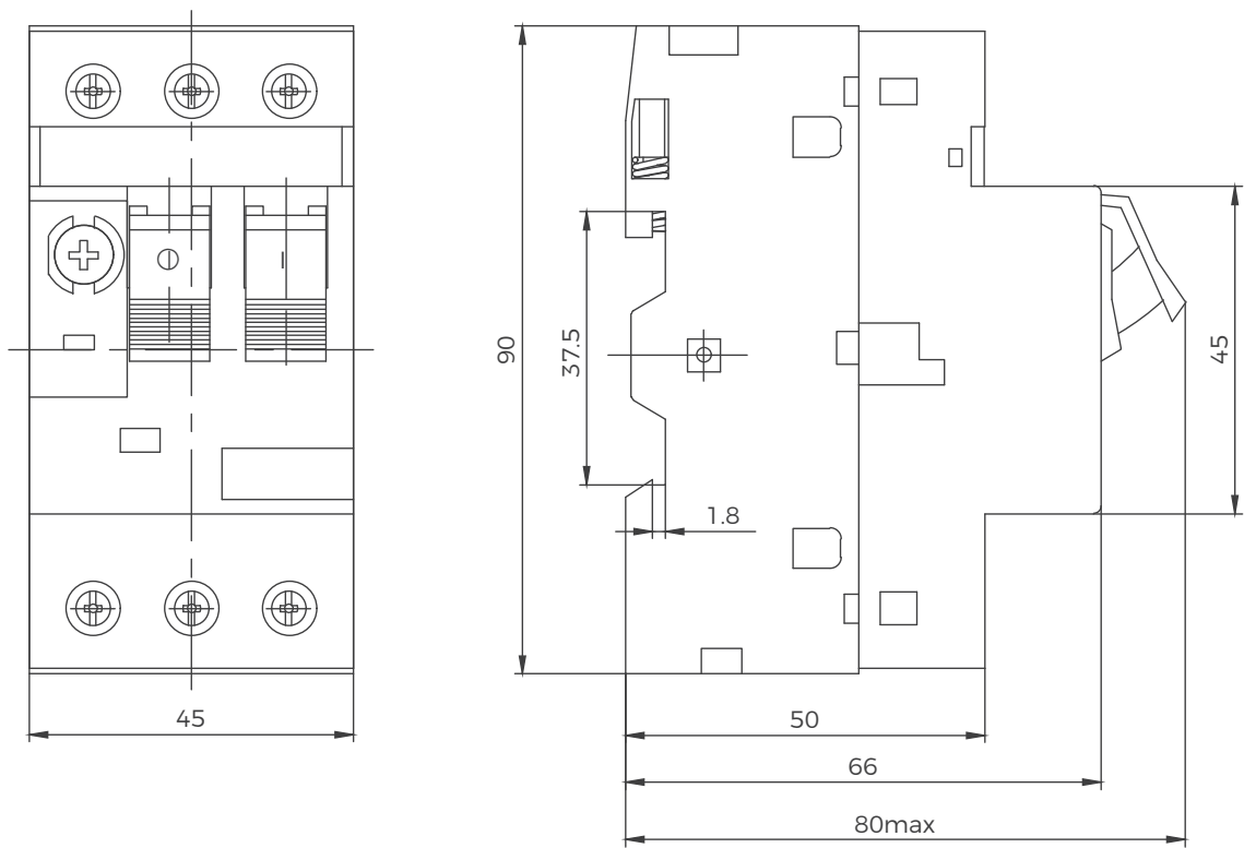
BD1-32 外形安装尺寸图
