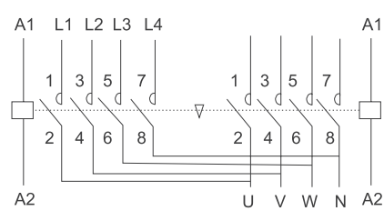
b. 控制双电源切换时接线图
