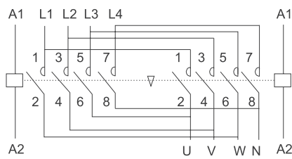
a. 控制可逆运转时接线图
