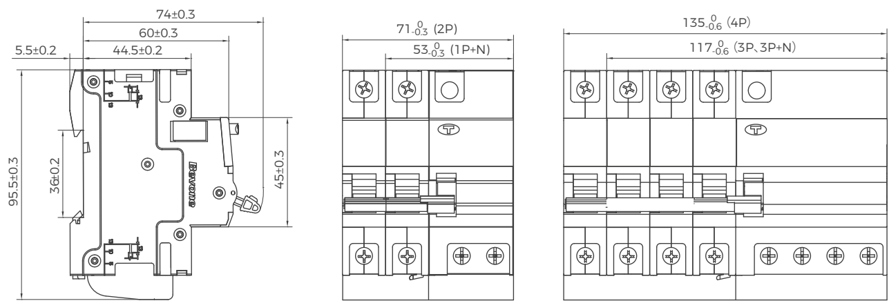
BB2L-63 外形尺寸
