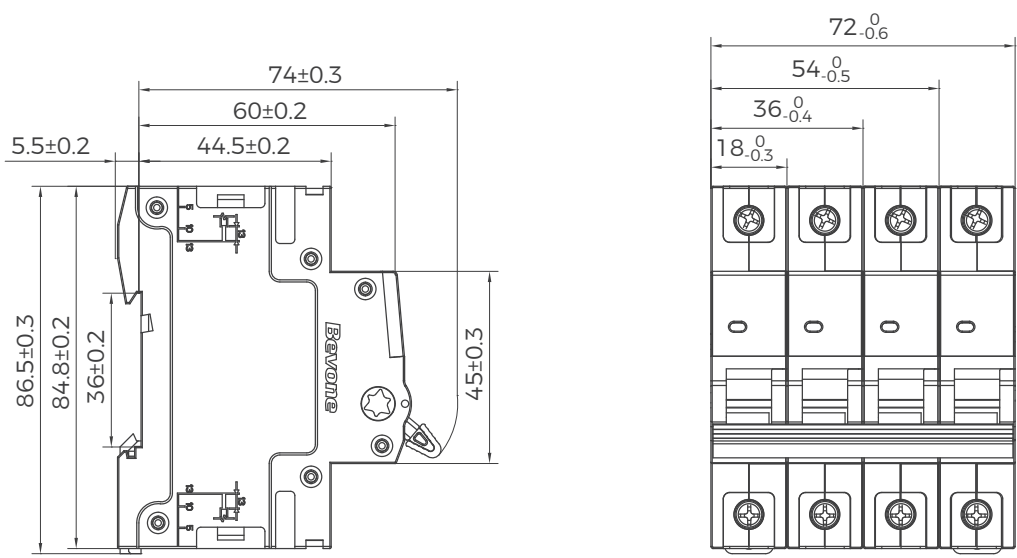
BB2G-125 外形尺寸
