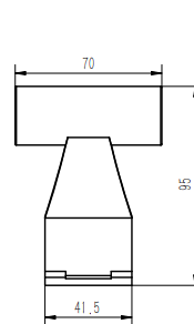
400-800 壳架加长手柄 外形尺寸图
