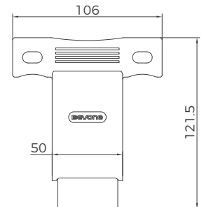
1600 壳架加长手柄 外形尺寸图
