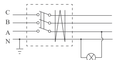
正确接线
