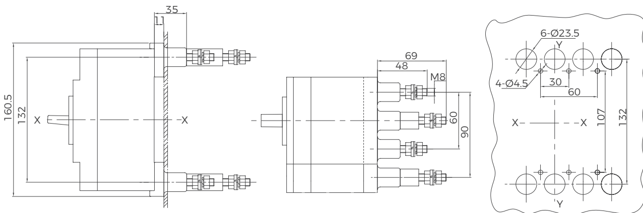
BM3E-125C/L/N/M/H 塑壳断路器板后接线
