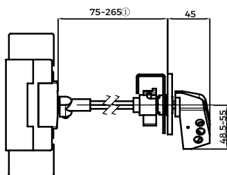
BG1-125 壳架柜外操作尺寸图
