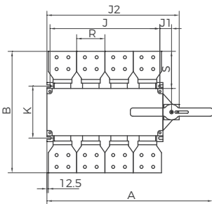
BG1Z1-3150A 正面直接操作
