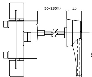
BG1-140~800 壳架柜外操作尺寸图
