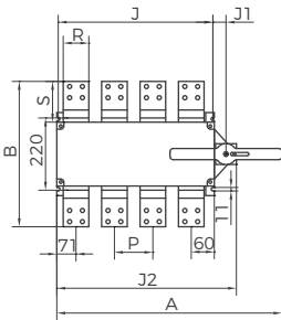
BG1Z1-2000~2500A 正面直接操作
