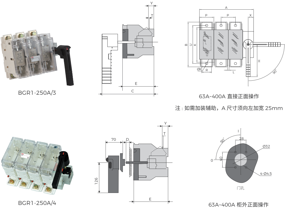
BCR1-63A~400A 正面操作隔离开关熔断器组外形与安装尺寸
