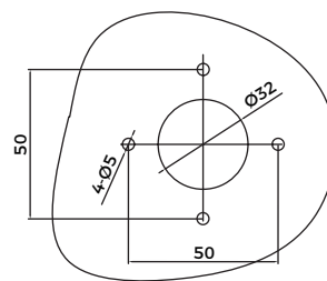
BG1-125 柜外操作开孔尺寸
