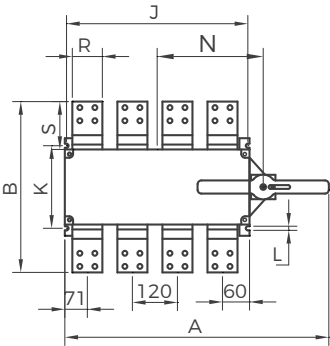
BG1C-2000~2500A 直接操作
