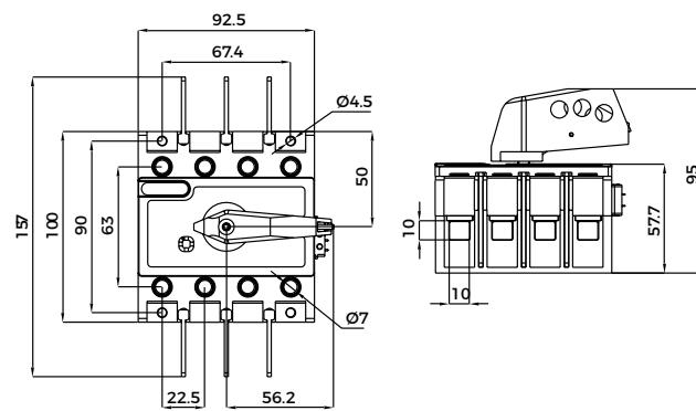
BG1-125 4P 直接安装尺寸图
