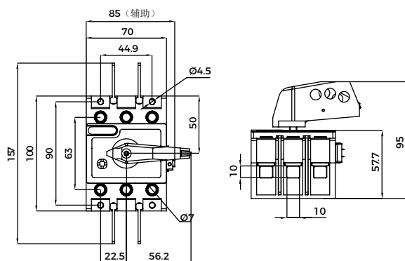
BG1-125 3P 直接安装尺寸图
