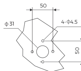
BG1-1000~3150 柜外面板开孔尺寸
