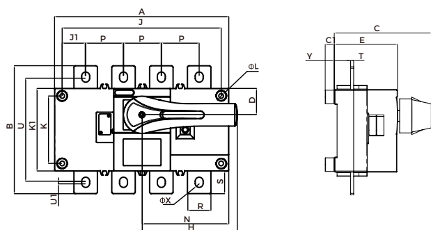
BG1-140-800 直接安装尺寸图
