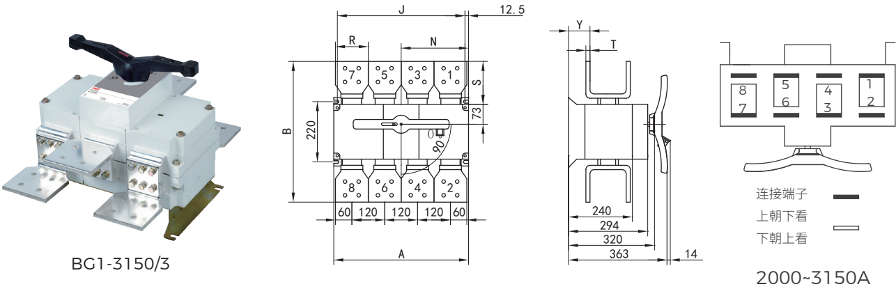
BG1-3150A 正面直接操作
