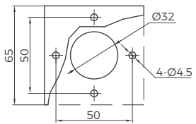
BC1-32~100 柜外面板开孔尺寸
