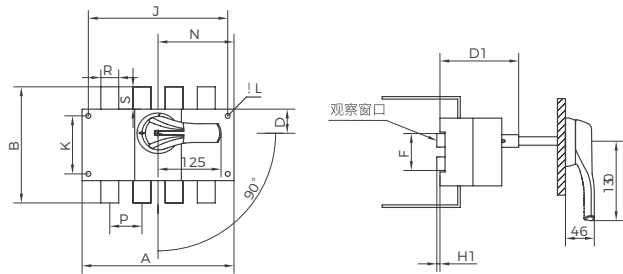
BG1-125~630A/B 柜外直接操作
