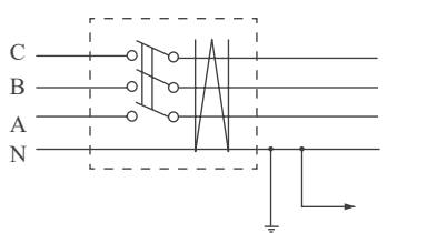
错误接线
