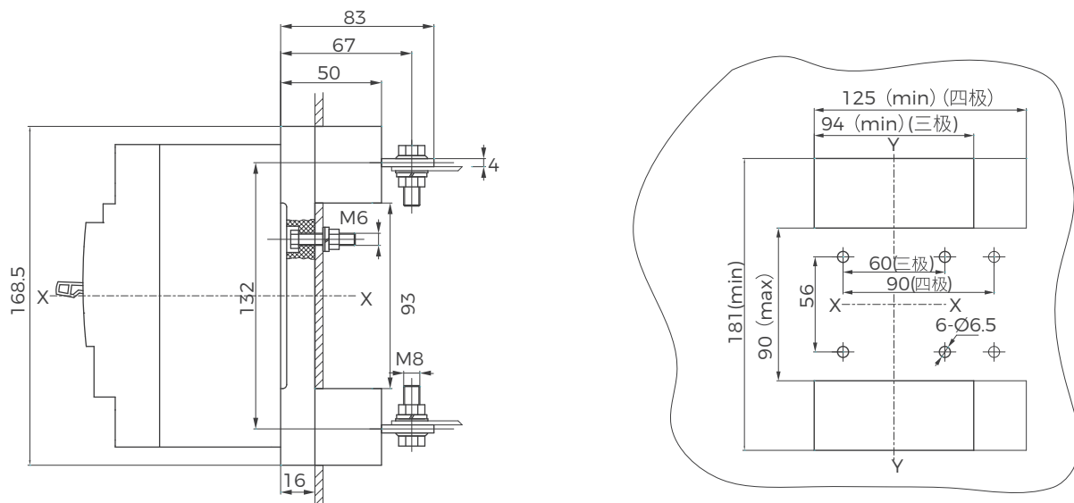
BM3E-125C/L/N/M/H 塑壳断路器插入式板后接线
