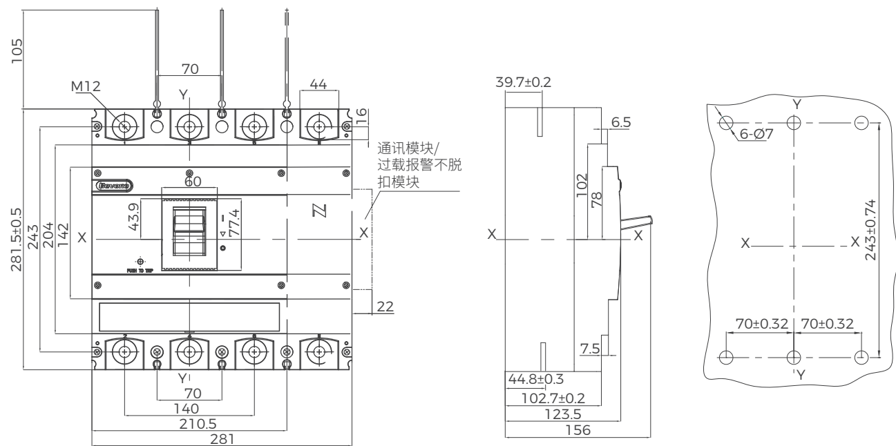
BM3E-800L/M/H 塑壳断路器板前接线
