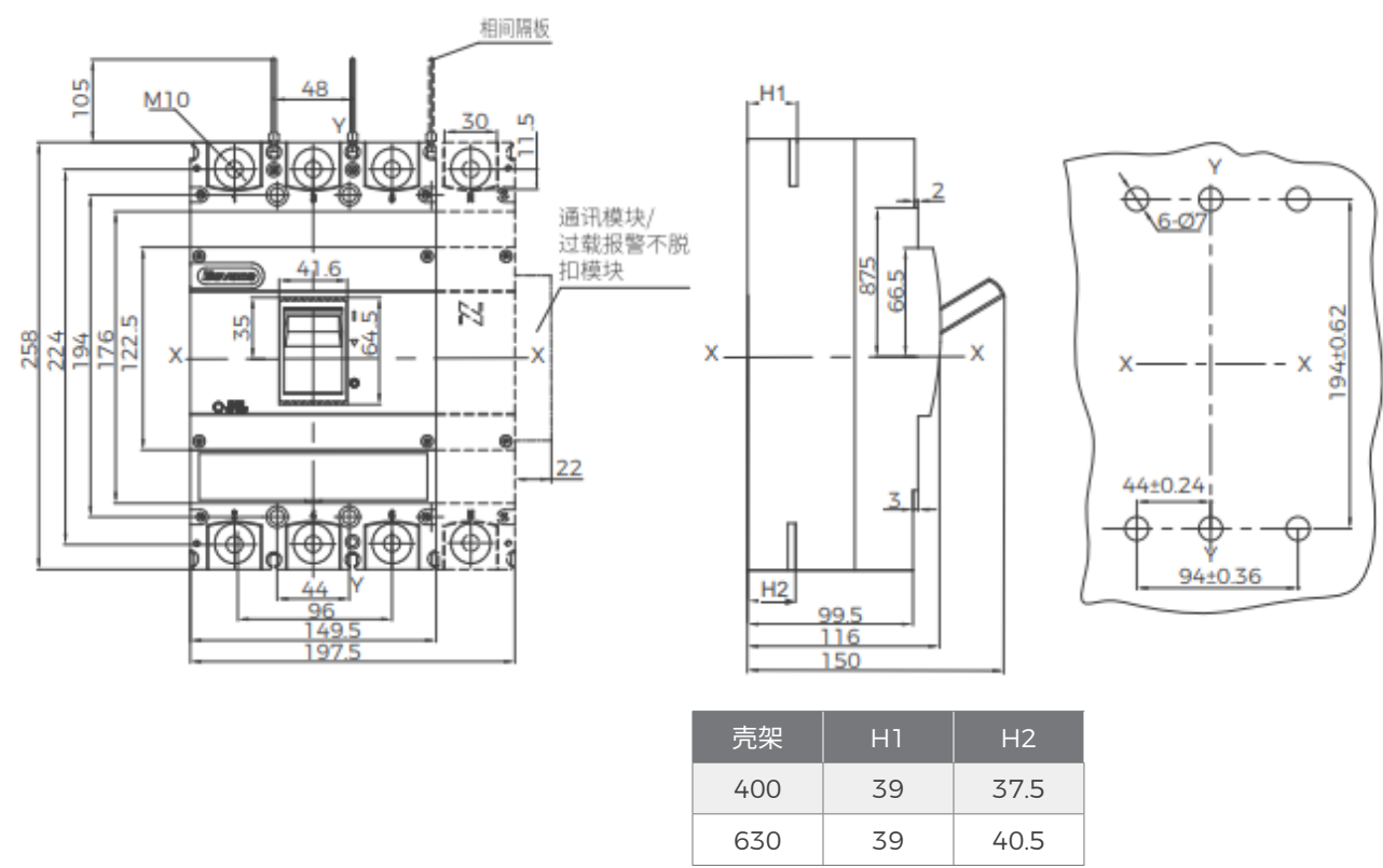
BM3E-400C/L/M/H、BM3E-630C/L/M/H 塑壳断路器板前接线
