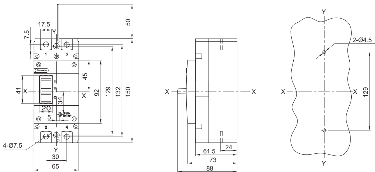
板前接线安装板开孔尺寸
