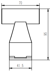
400-800 壳架加长手柄 外形尺寸图
