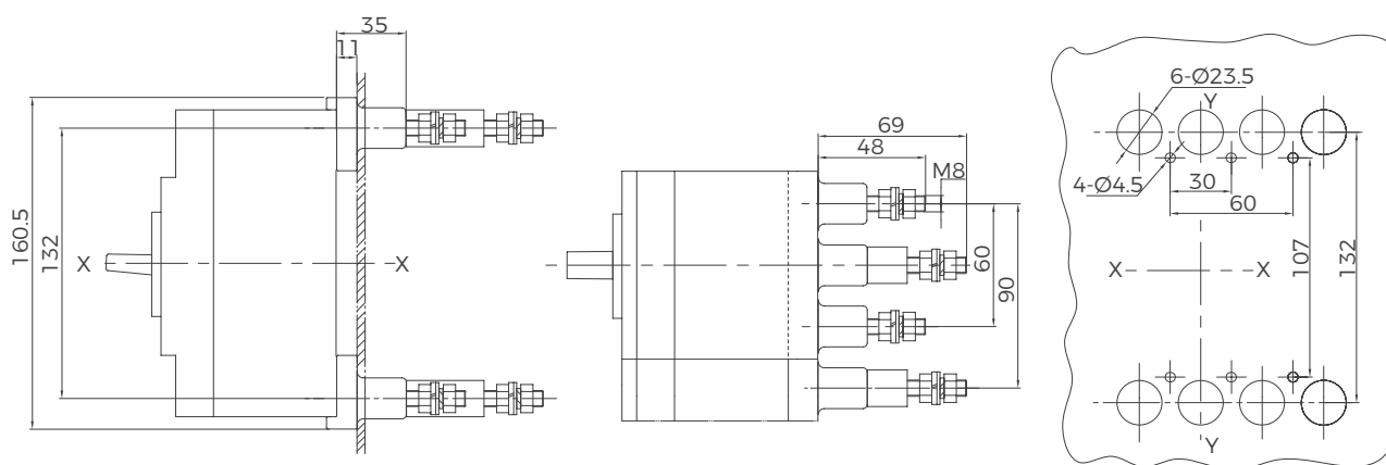
BM3E-125C/L/N/M/H 塑壳断路器板后接线
