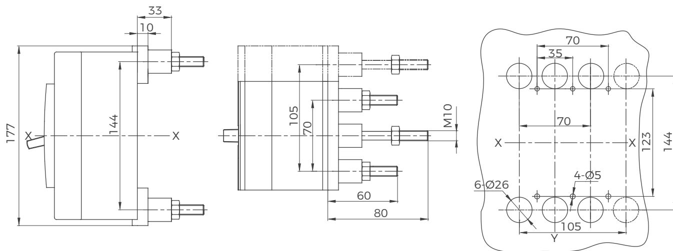
BM3-250 (C、L、F、N、M、S、H) 插入式板后接线 ( 三极、四极 )
