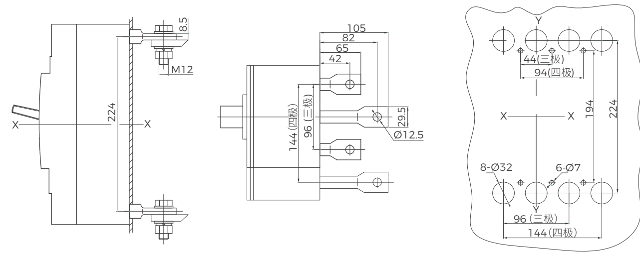
BM3E-400C/L/M/H、BM3E-630C/L/M/H 塑壳断路器板后接线
