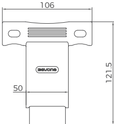
1600 壳架加长手柄 外形尺寸图
