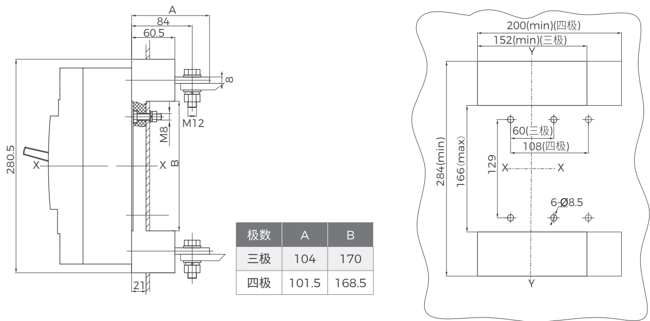
BM3E-400C/L/M/H、BM3E-630C/L/M/H 塑壳断路器插入式板后接线
