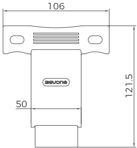
1600 壳架加长手柄 外形尺寸图
