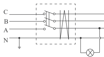
正确接线
