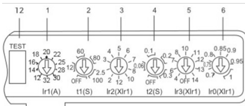
BM3E-125, In=32A 电子式脱扣器
