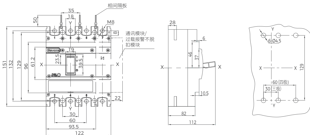
BM3E-125C/L/N/M/H 塑壳断路器板前接线
