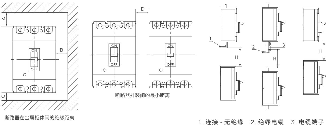
BM3 系列塑料外壳式断路器安全距离 (mm)
