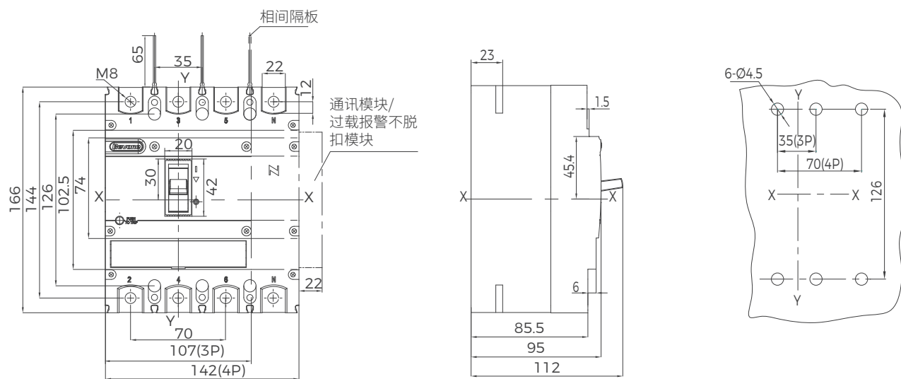
BM3E-250C/L/M/H 塑壳断路器板前接线
