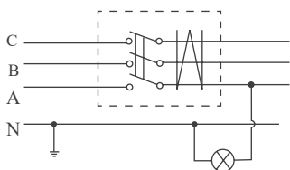
错误接线
